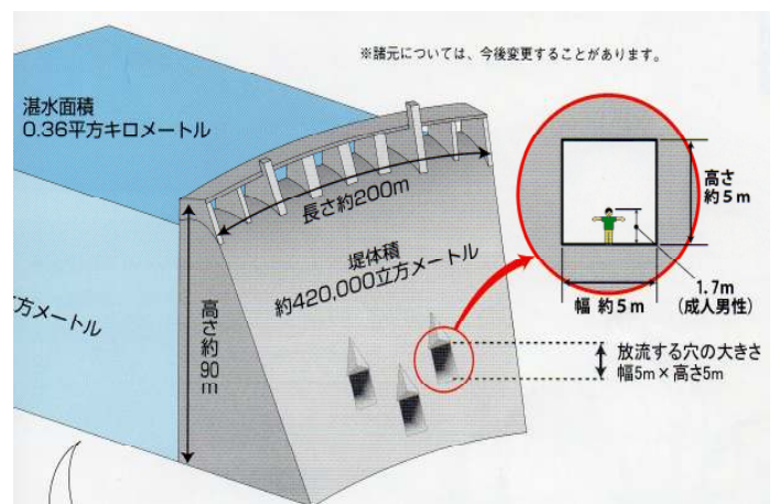
立野ダムの「穴」は5m×5m(国交省資料より)
