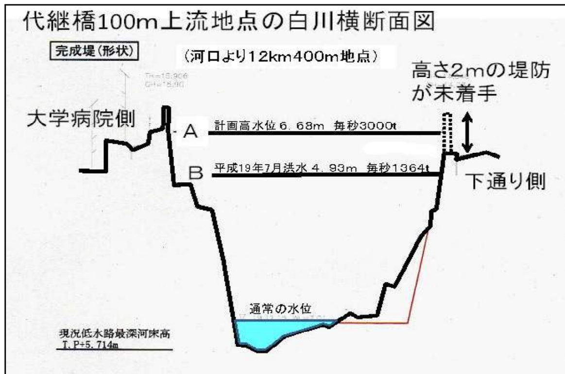
白川の水位と流量(A, Bで表示)
