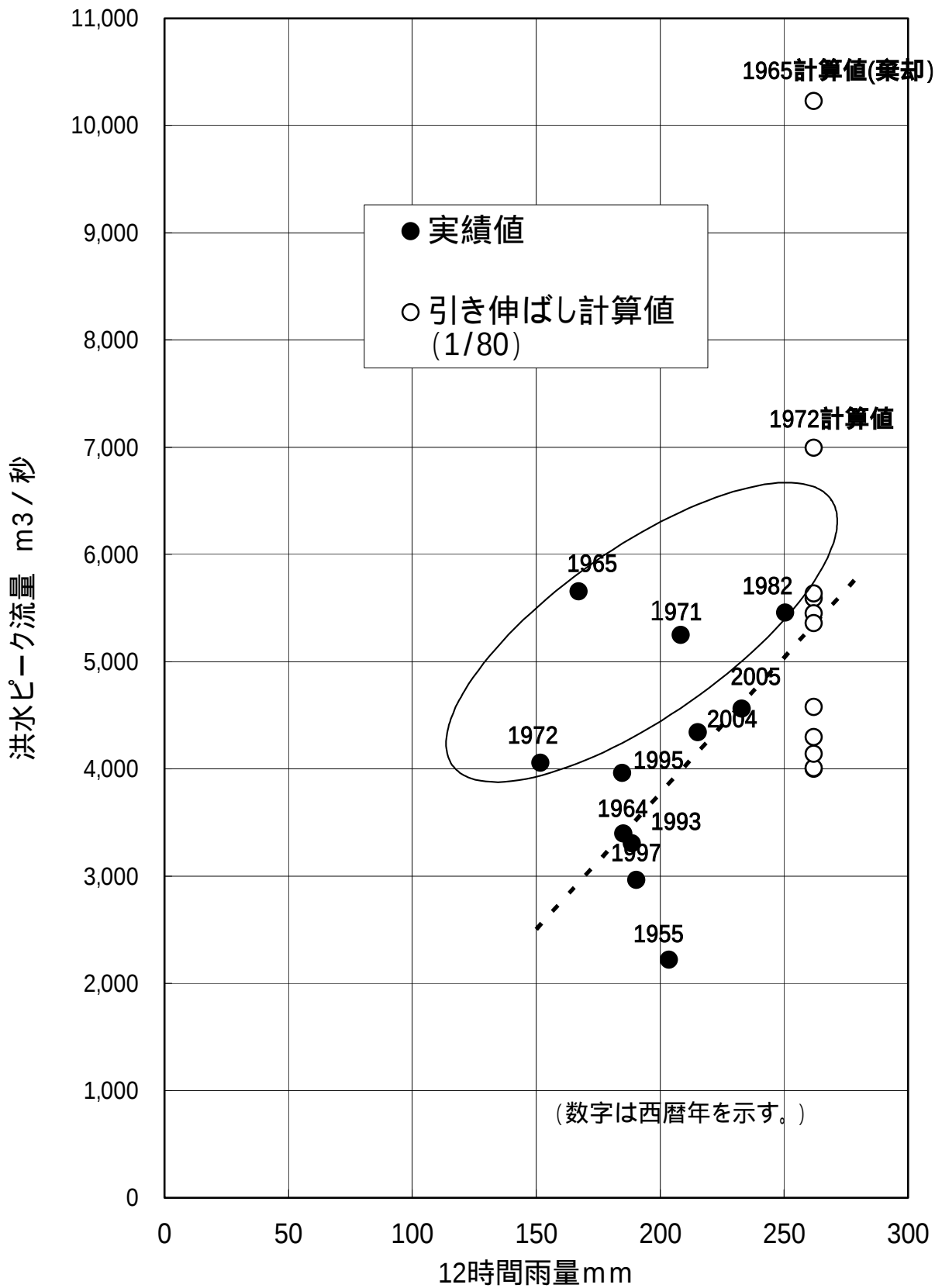
図1 降雨量と洪水ピーク流量の関係(人吉)
