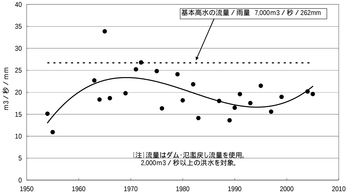
図2 球磨川人吉地点の〔年最大洪水ピーク流量〕 / 〔その洪水時の12時間最大雨量〕
